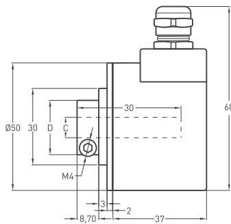
半空轴型
