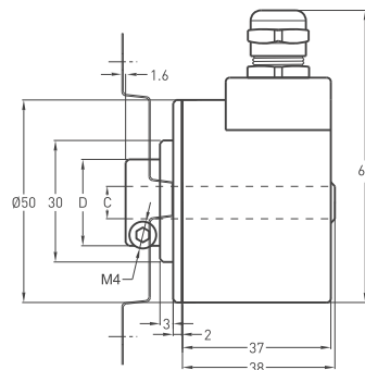
全空轴型
