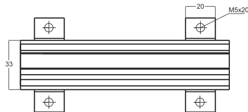
MP2 铝轨
